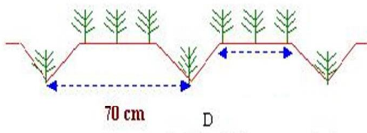
شکل ۲۲ - در هنگام کشت بر روی پشته با تناوب ، گندم، جو و کلزا باید دقت کرد که درون جویها چیزی کاشته نشود
