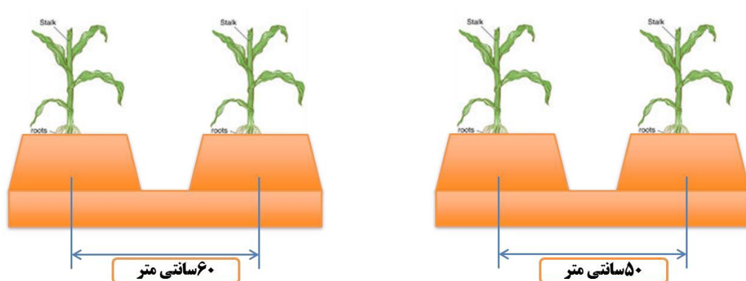
شکل ۱۹- سایر الگوهای قابل حصول کاشت گندم در پشته های بلند در تناوب با ذرت علوفه ای که ماشین برای آنها موجود است
