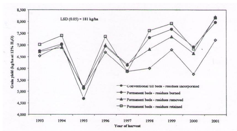
شکل ۱۱- تاثیر مدیریت بقایای گیاهی و خاک‌ورزی بر عملکرد گندم (Sayre, 2000)
